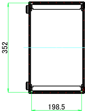
B-B ( 1 : 8.5 )
