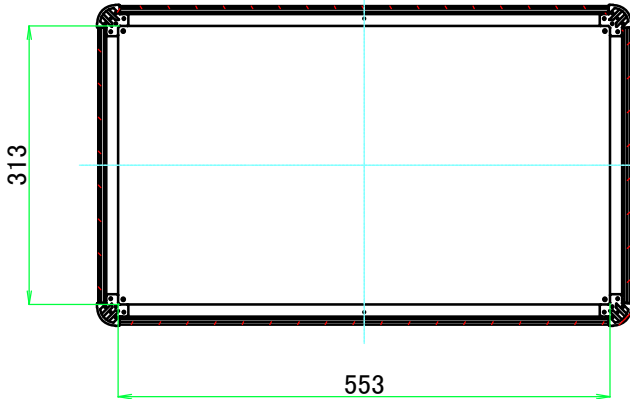
C-C ( 1 : 8.5 )
