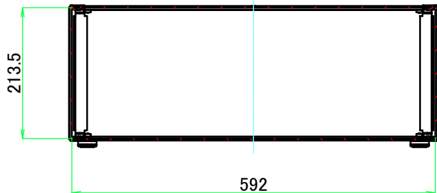
A-A ( 1 : 8.5 )
